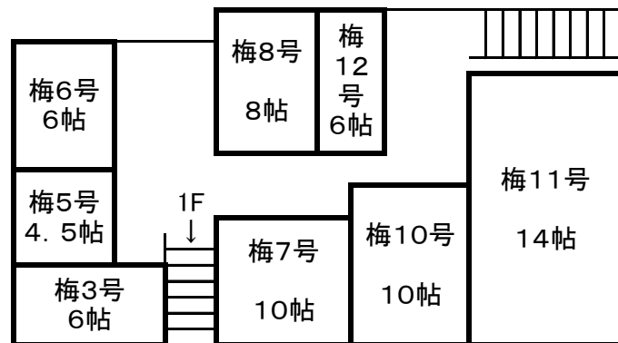
富士屋旅館 旧館2F見取り図
